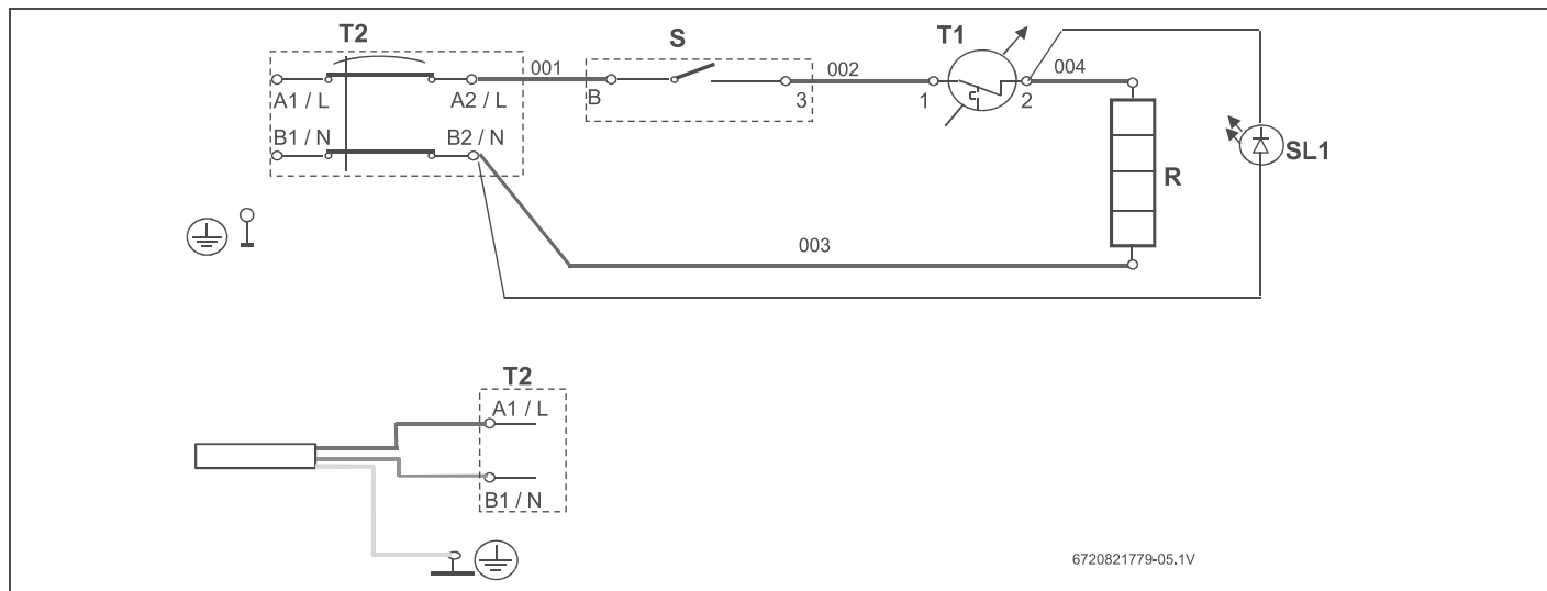
Rys. 5 Schemat połączeń
