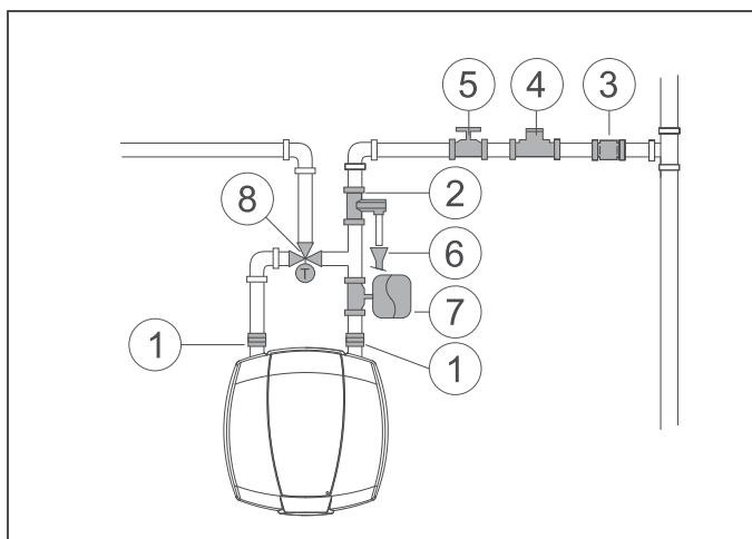
Rys. 10 Przyłącze wody
