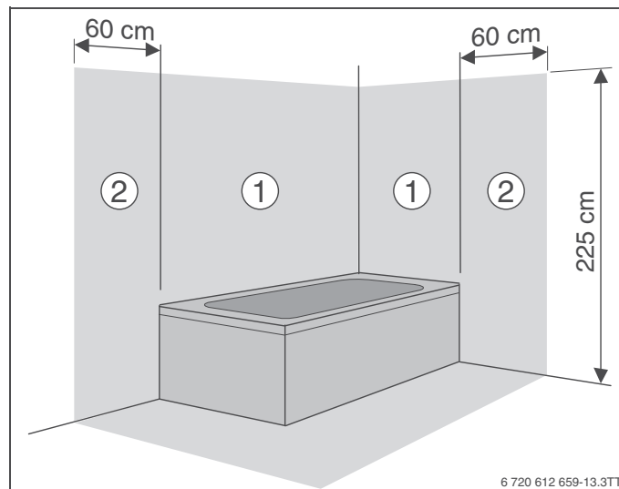
Rys. 6 Strefy ochronne
