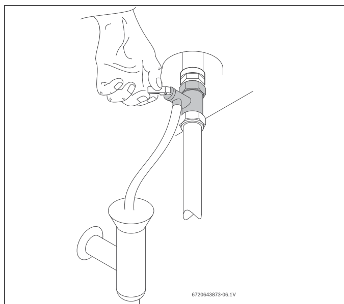
Rys. 12 Ręczne otwieranie zaworu bezpieczeństwa
