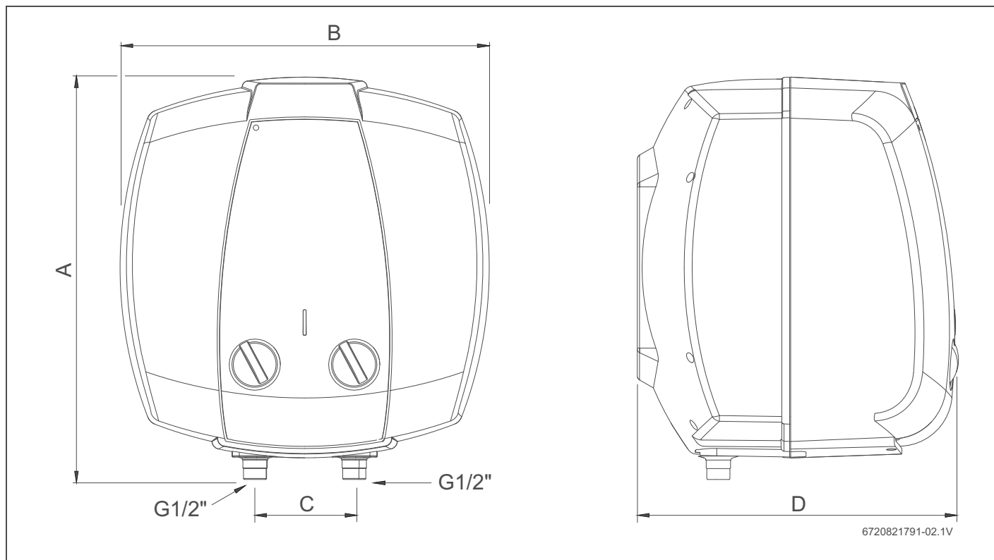
Rys. 2 Wymiary w mm (montaż ścienny)
