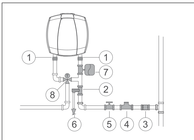
Rys. 9 Przyłącze wody
