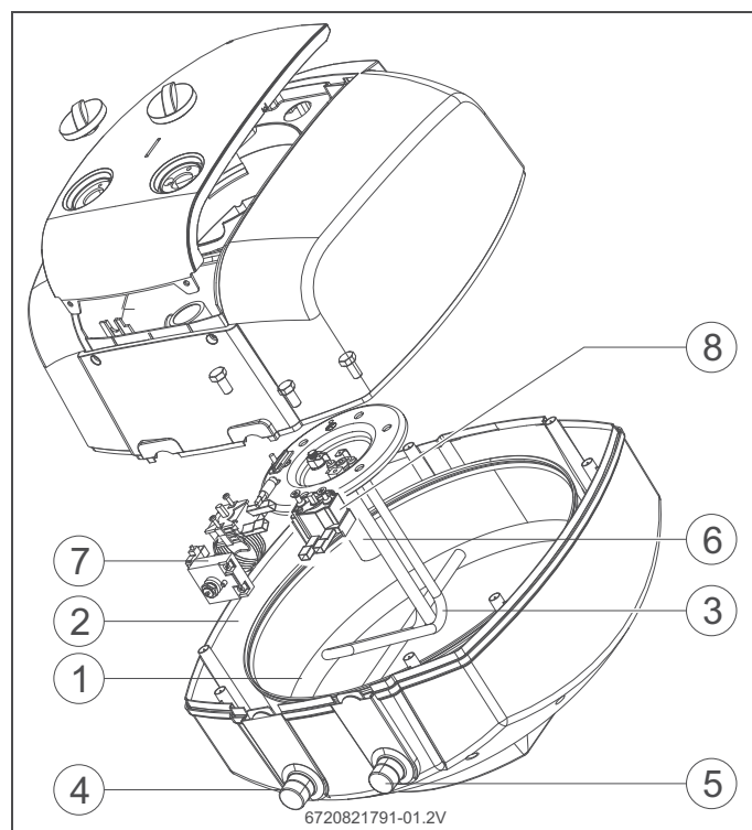
Rys. 4 Konstrukcja
