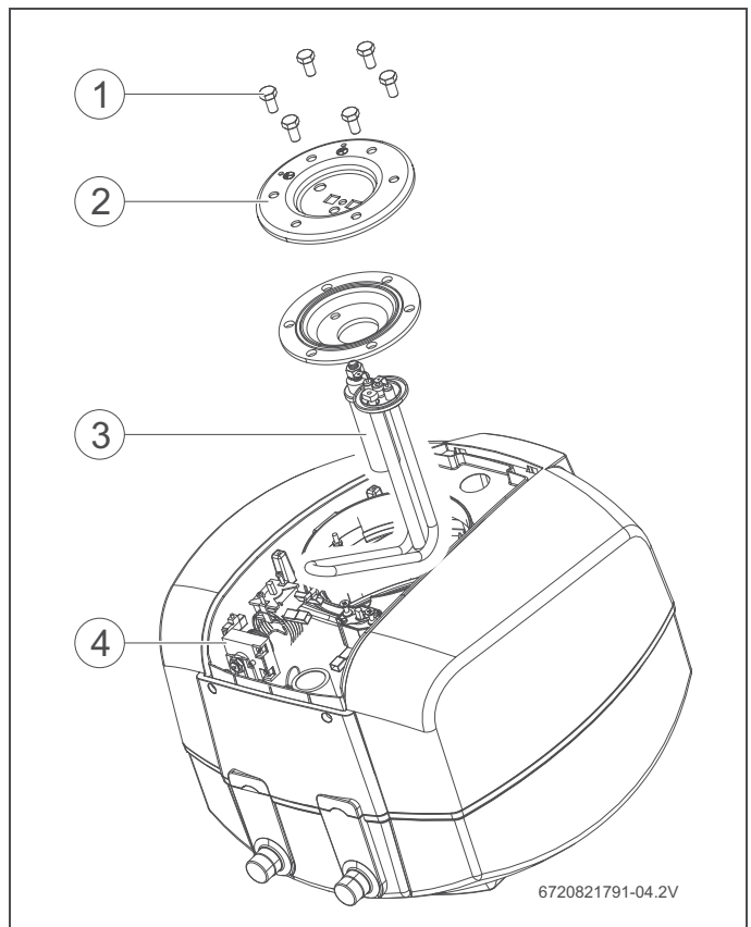
Rys. 14 Dostęp do wnętrza urządzenia i oznaczenie elementów
