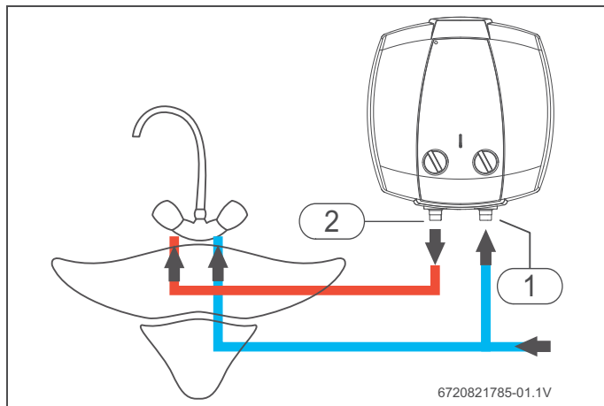
Rys. 7 Instalacja nad umywalką
