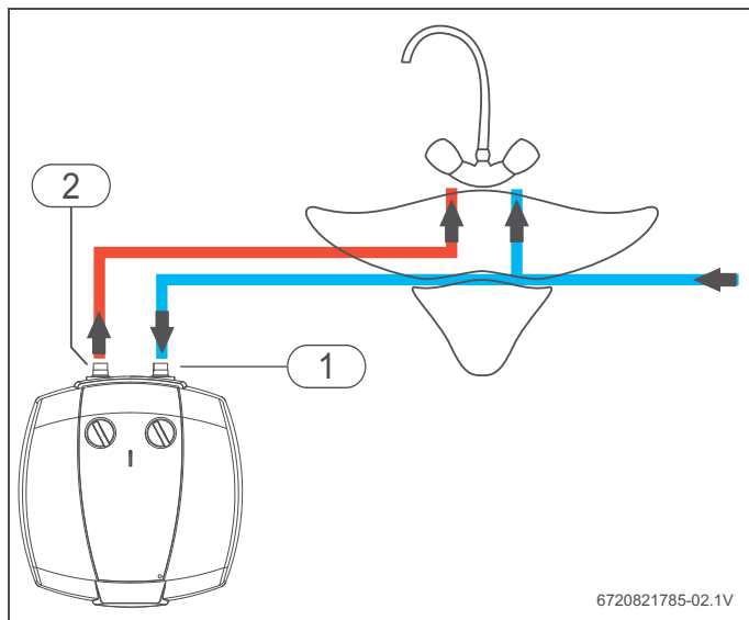
Rys. 8 Instalacja pod umywalką
